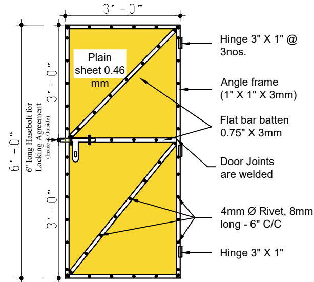
Door Elevation
